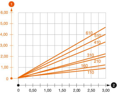
Diagrama de carga escuadra tipo AS 30
