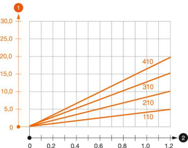
Diagrama de carga escuadra tipo MWAM 12
