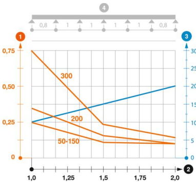
Diagrama de carga bandeja de rejilla GR-Magic tipo GRM 35
