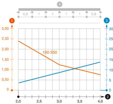
Diagrama de carga bandeja de chapa SKS 110
