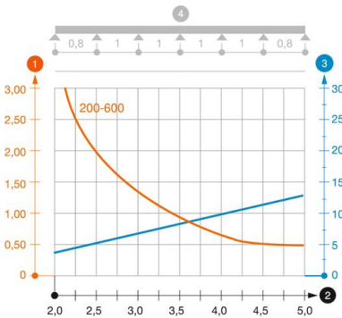
Diagrama de carga bandeja de escalera tipo LG 110 VS
