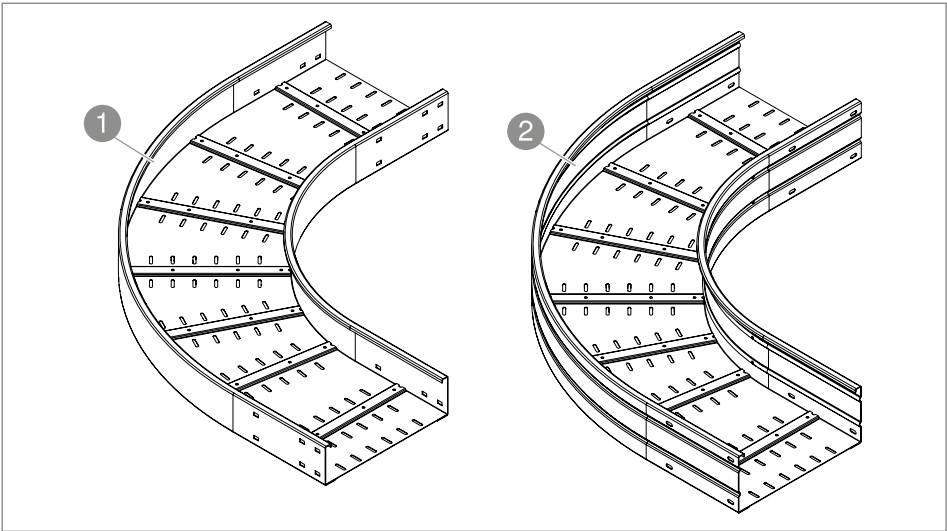
Fig. 4: 90° bends
