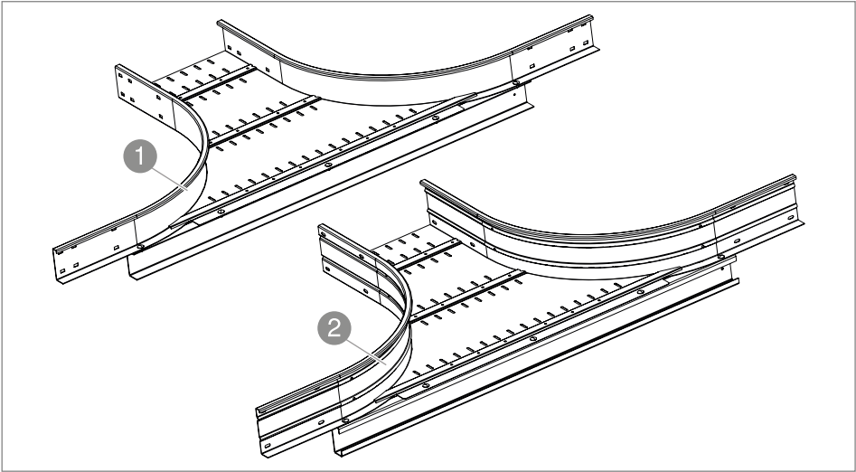
Fig. 6: Add-on tees
